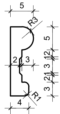
LAJSNA MJ 1:5
