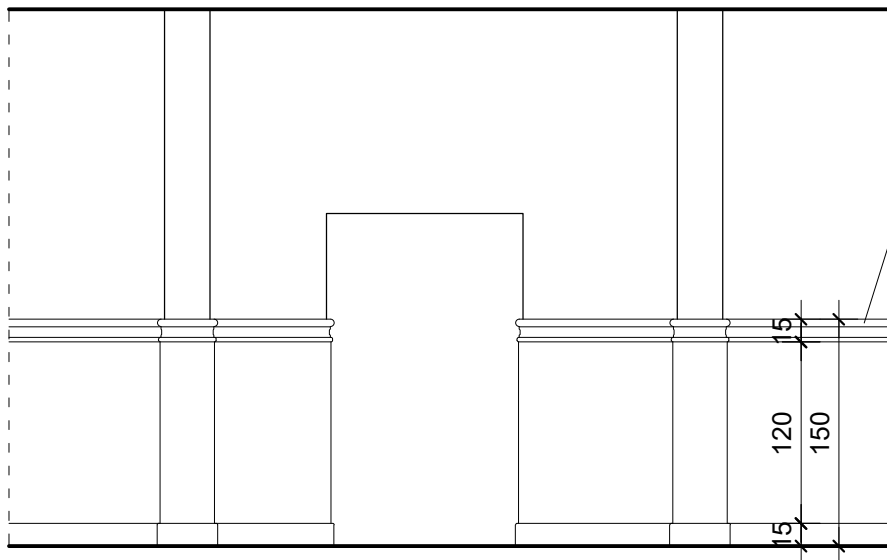
POGLED 2
