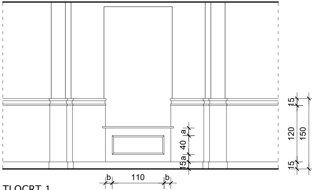
TLOCRT 1
