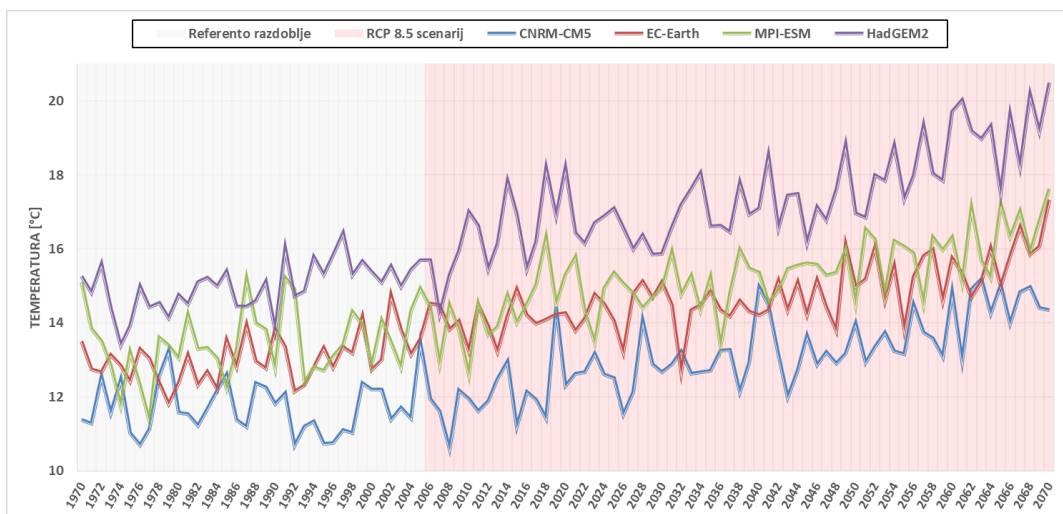
Slika 8.2-3 Vremenski niz srednje maksimalne godišnje temperature (°C) za Grad Crikvenicu za četiri integracije RegCM modelom. Izvor podataka: DHMZ
