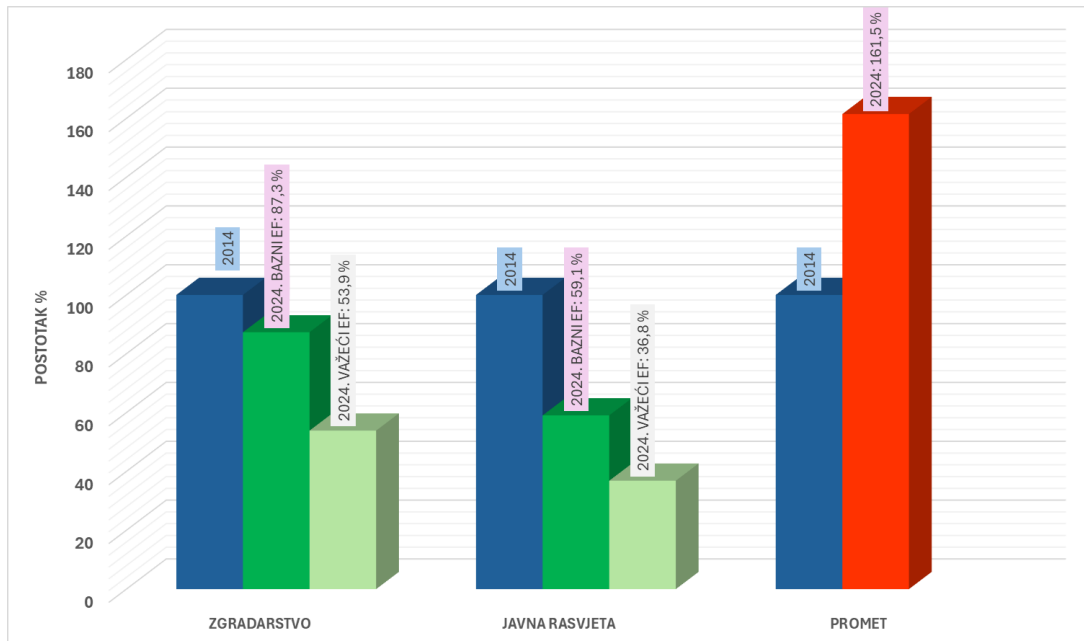
Slika 6.4-1 Emisije stakleničkih plinova u referentnom i kontrolnom stanju po sektorima s prikazom postotne promjene
