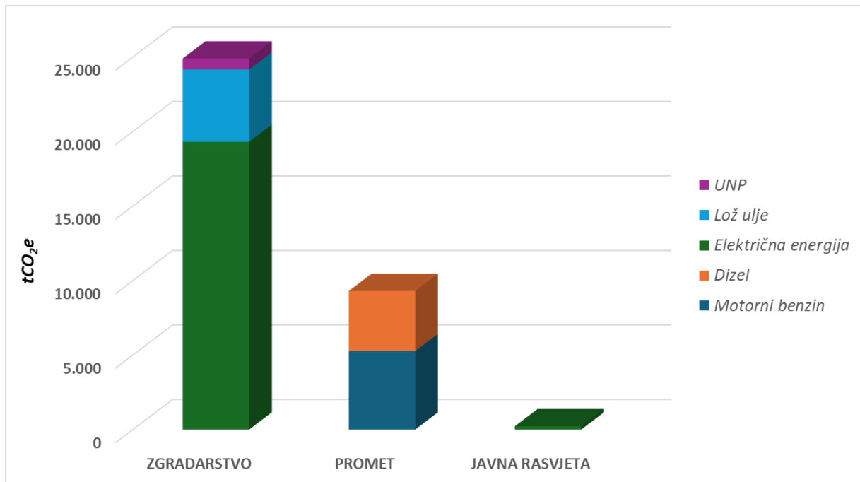
Slika 5.4-1 Ukupne emisije stakleničkih plinova po sektorima i energentima u referentnoj 2014. godini na području Grada Crikvenice (tCO 2 e)
