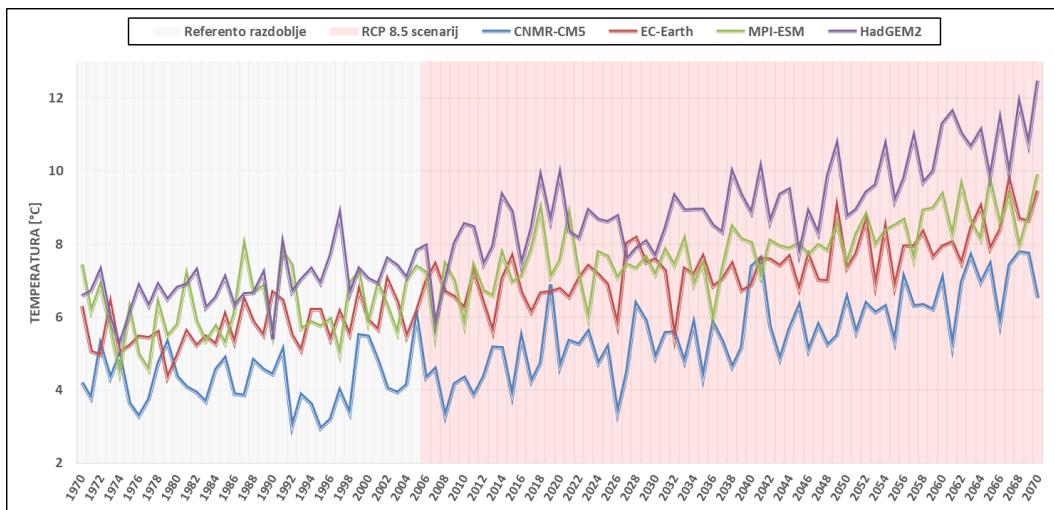
Slika 8.2-2 Vremenski niz srednje minimalne godišnje temperature (°C) za Grad Crikvenicu za četiri integracije RegCM modelom. Izvor podataka: DHMZ
