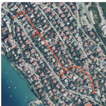
Trasa nove vodoopskrbne mreže
