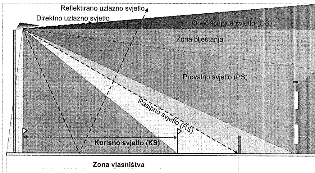
Slika 3 Korisno i štetno svjetlo javne rasvjetel III
